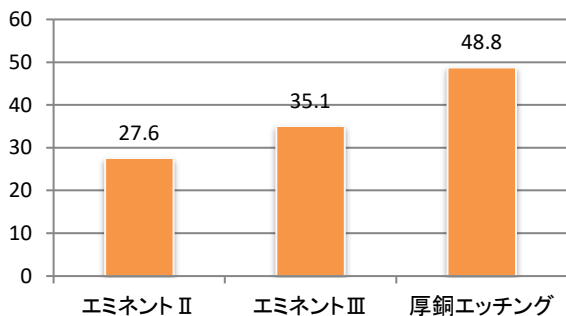
エッチングレート (um/min)
